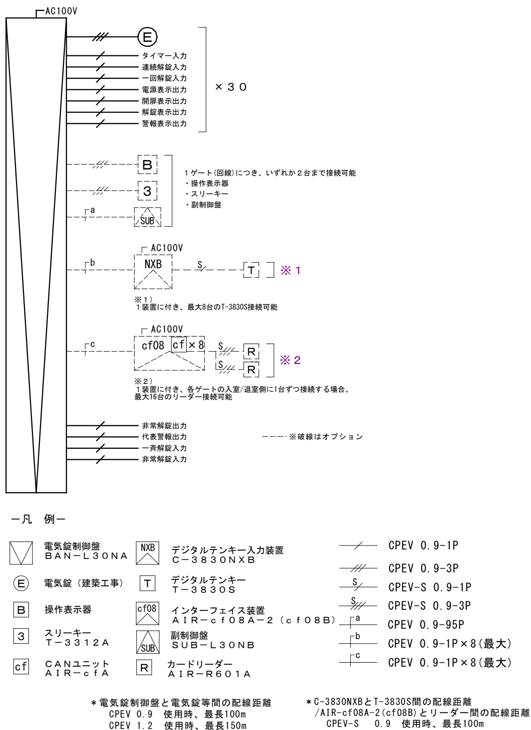
図6-1. 系統図
