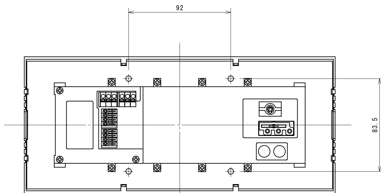
背面図
