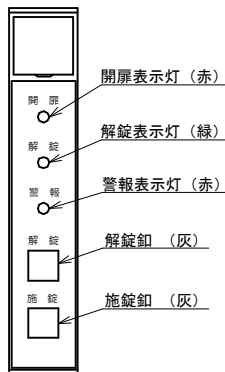
選択パネル詳細 (4:1) 繰り返しモード用パネル使用時
