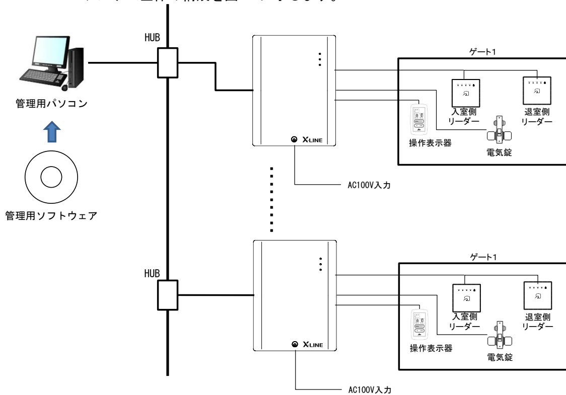
図2-2 システム全体の構成
