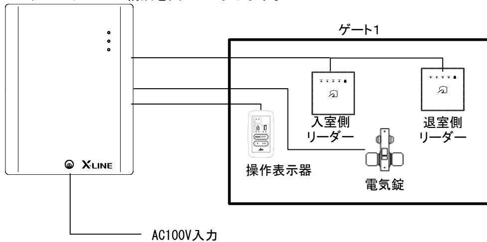
図2-1 スタンドアロンの構成
