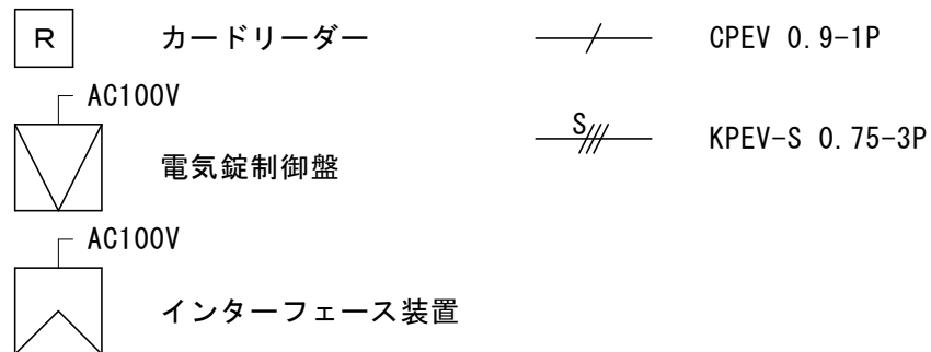
図3 インターフェース装置使用時系統図
