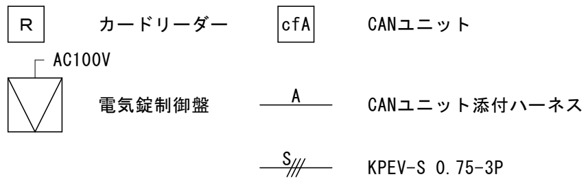
図2 CANユニット盤内搭載時系統図
