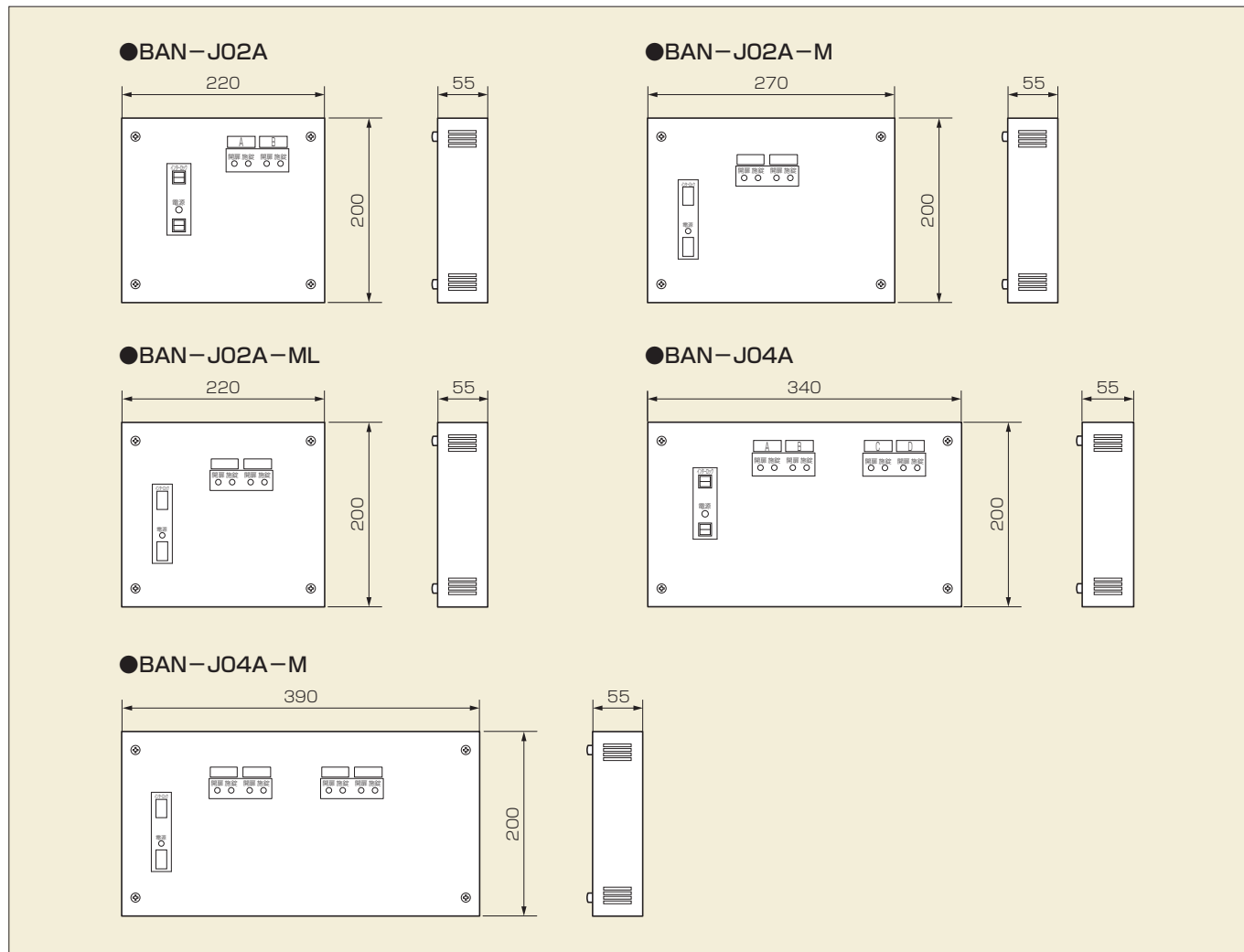
外形図(単位:mm)
