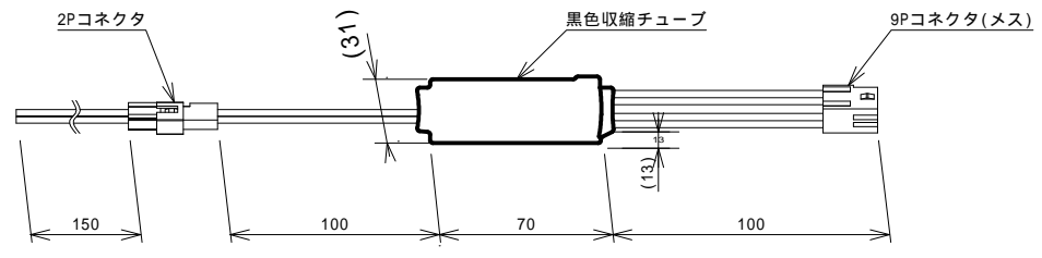
電気錠アダプター：同梱品×1個 縮尺1:3
