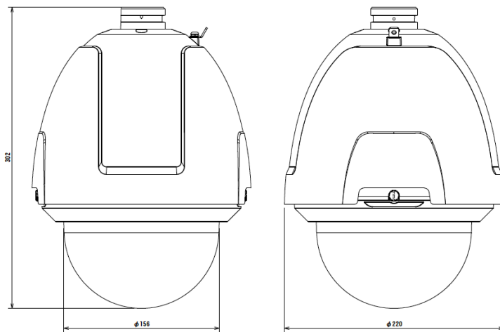
PTZドームカメラ Z-2PTZD
