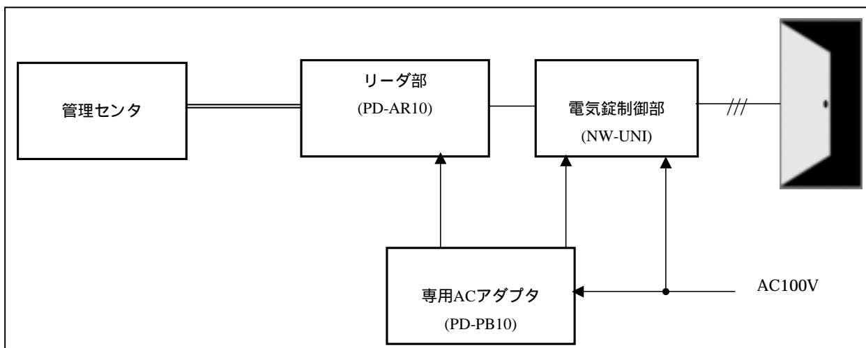
システム構成:管理センター・電気錠制御部・電源部・リーダ部 ( F e l i C a 方式、 E d y 対応)
